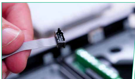
3. IL CAVO flat permette di collegare facilmente tutti i moduli e di configurarli automaticamente in caso di sostituzione
